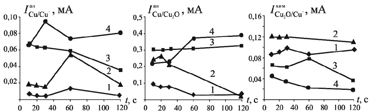
Рис. 5. Зависимости тока активного растворения меди I_{\text{Cu/Cu}^+}^{\text{ан}} , тока образования оксида I_{\text{Cu/Cu}_2\text{O}}^{\text{ан}} и его химического растворения I_{\text{Cu}_2\text{O/Cu}^+}^{\text{хим}} от времени при E_D = -0,17 (1), -0,05 (2), 0,10 (3) и 0,20 В (4)
